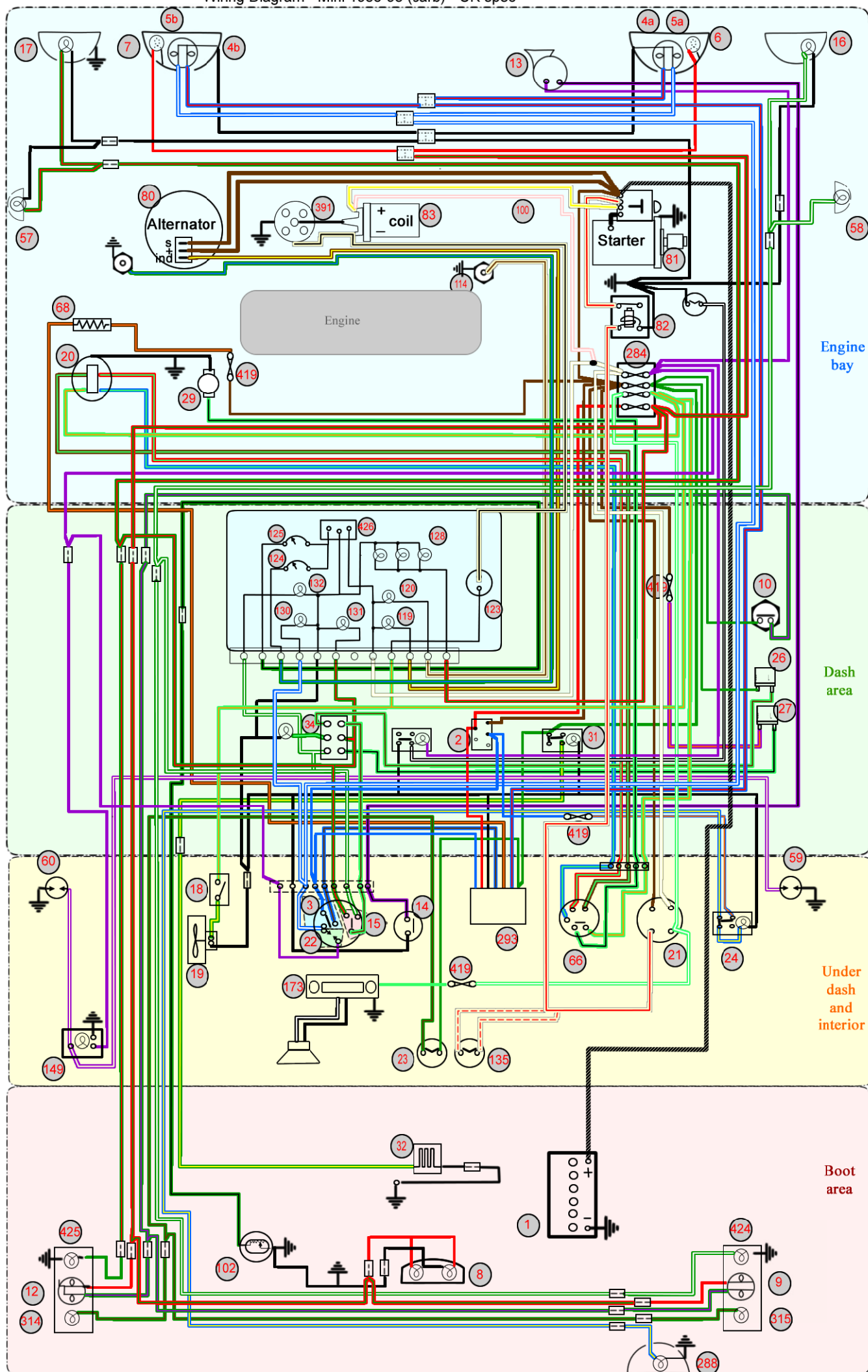
Wiring Diagram - Mini 1988-93 (carb) - UK spec
